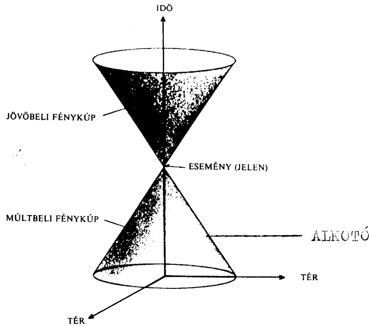
3. ábra A fénykúp keletkezésének módja /S.Hawking/
